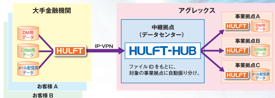
図 HULFT-HUBによるBPOのデータ連携基盤
