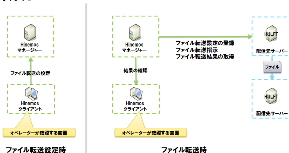
ファイル転送設定時とファイル転送時の Hinemos-HULFT 間通信
