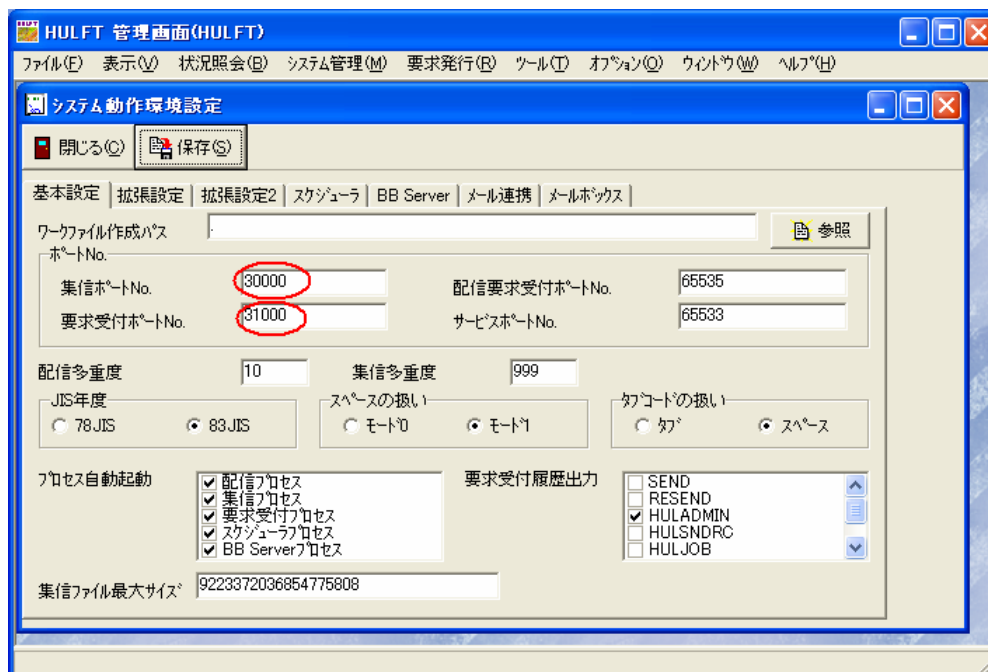
画面 2-1 システム動作環境設定画面「基本設定」タブ
