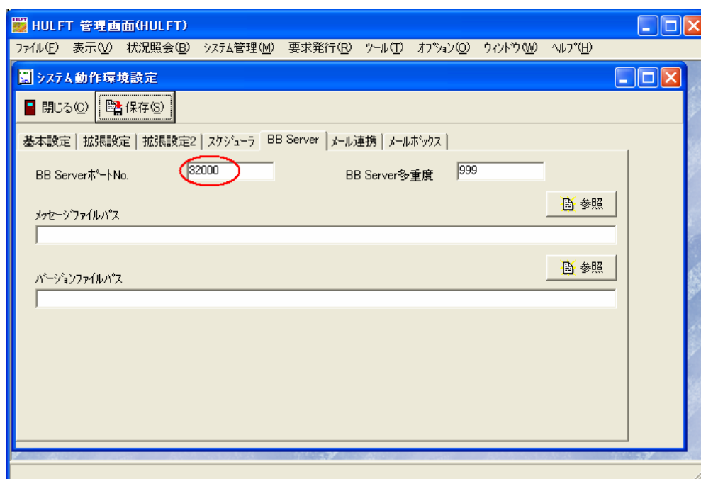
画面 3-1 システム動作環境設定画面「BB Server」タブ
